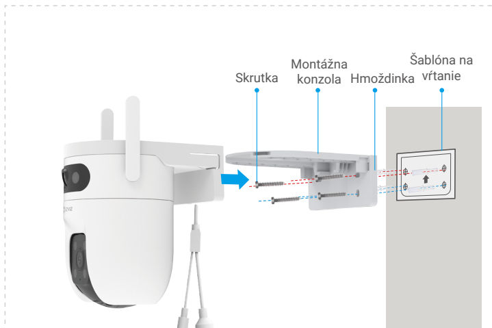
Obr. 2 Nástenné upevnenie
