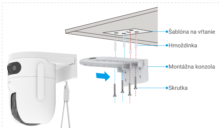
Obr. 1 Stropné upevnenie
